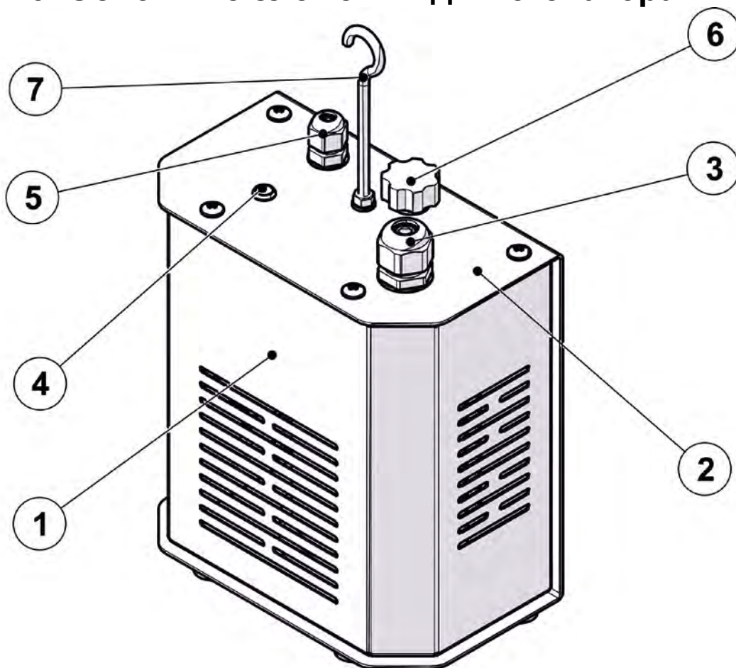
Рис. 3 Основные элементы дымогенератора
